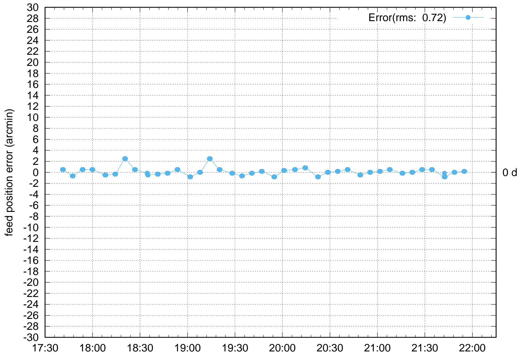
FPS Rotation error: C13-NEW-FPS 08Feb2022
