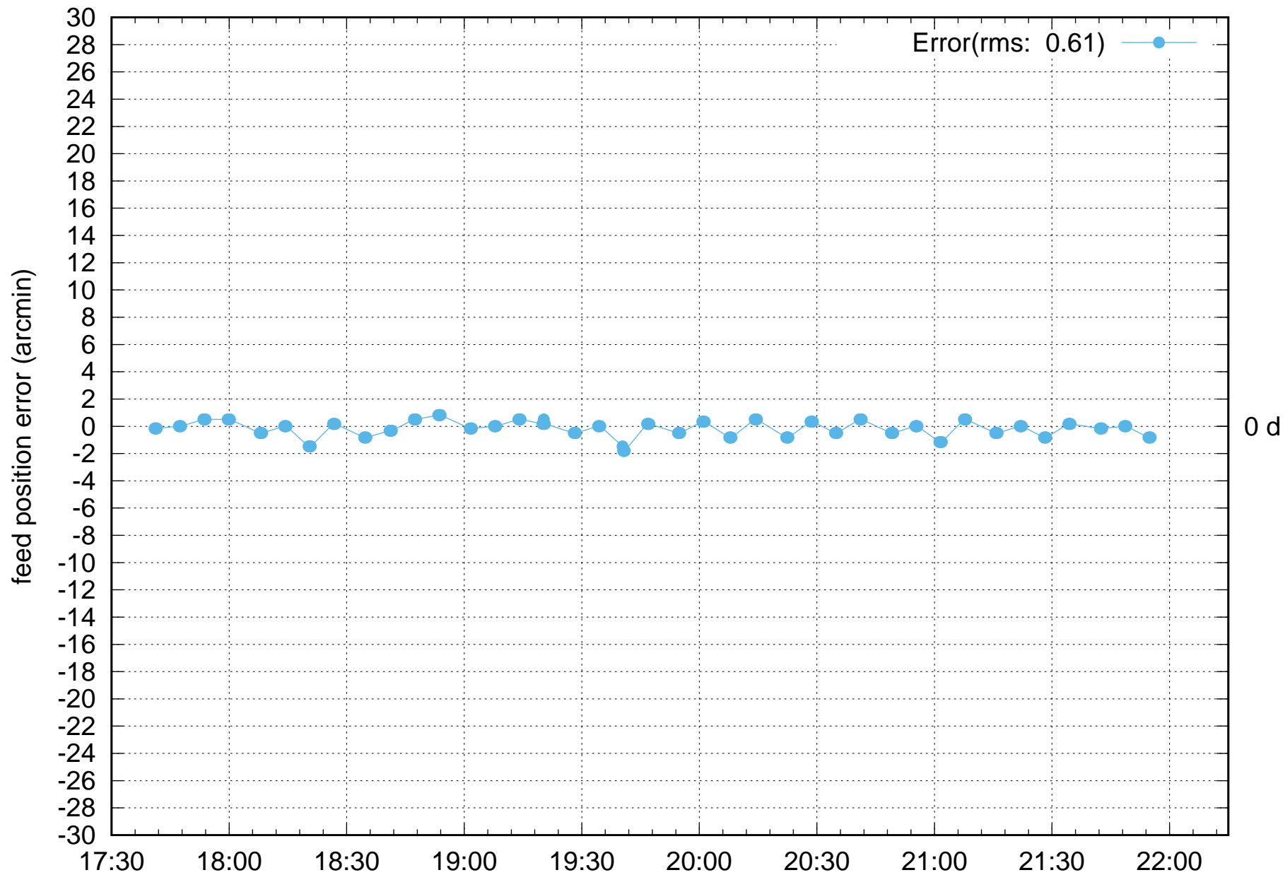
FPS Rotation error: C09-NEW-FPS 08Feb2022
