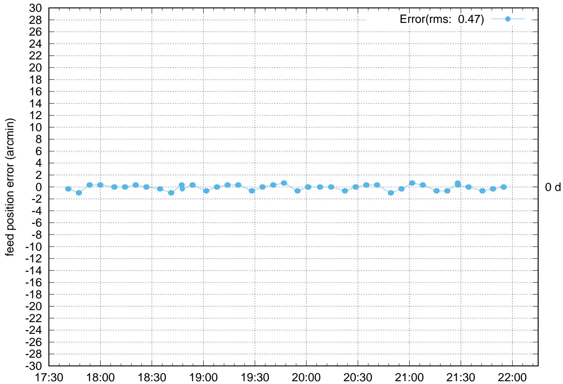
FPS Rotation error: C01-NEW-FPS 08Feb2022
