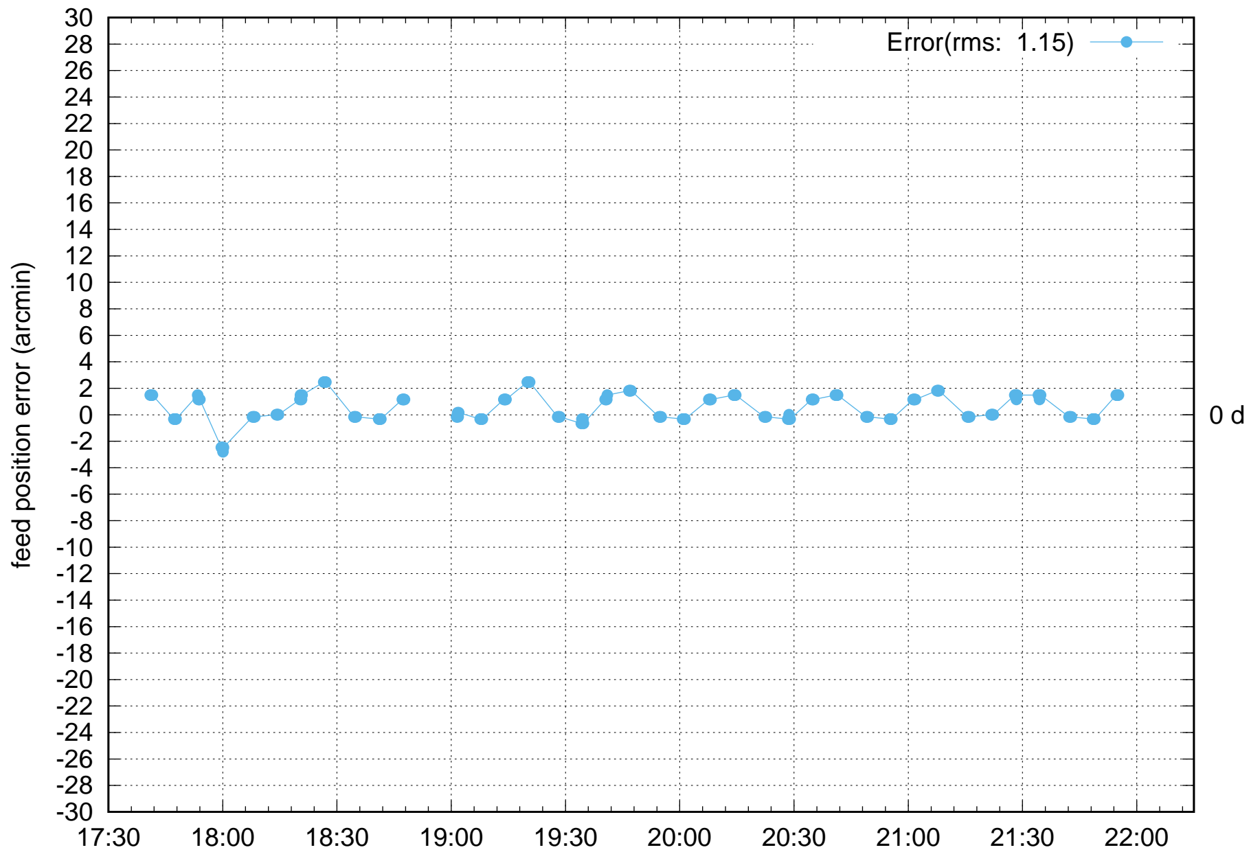
FPS Rotation error: W05-NEW-FPS 08Feb2022
