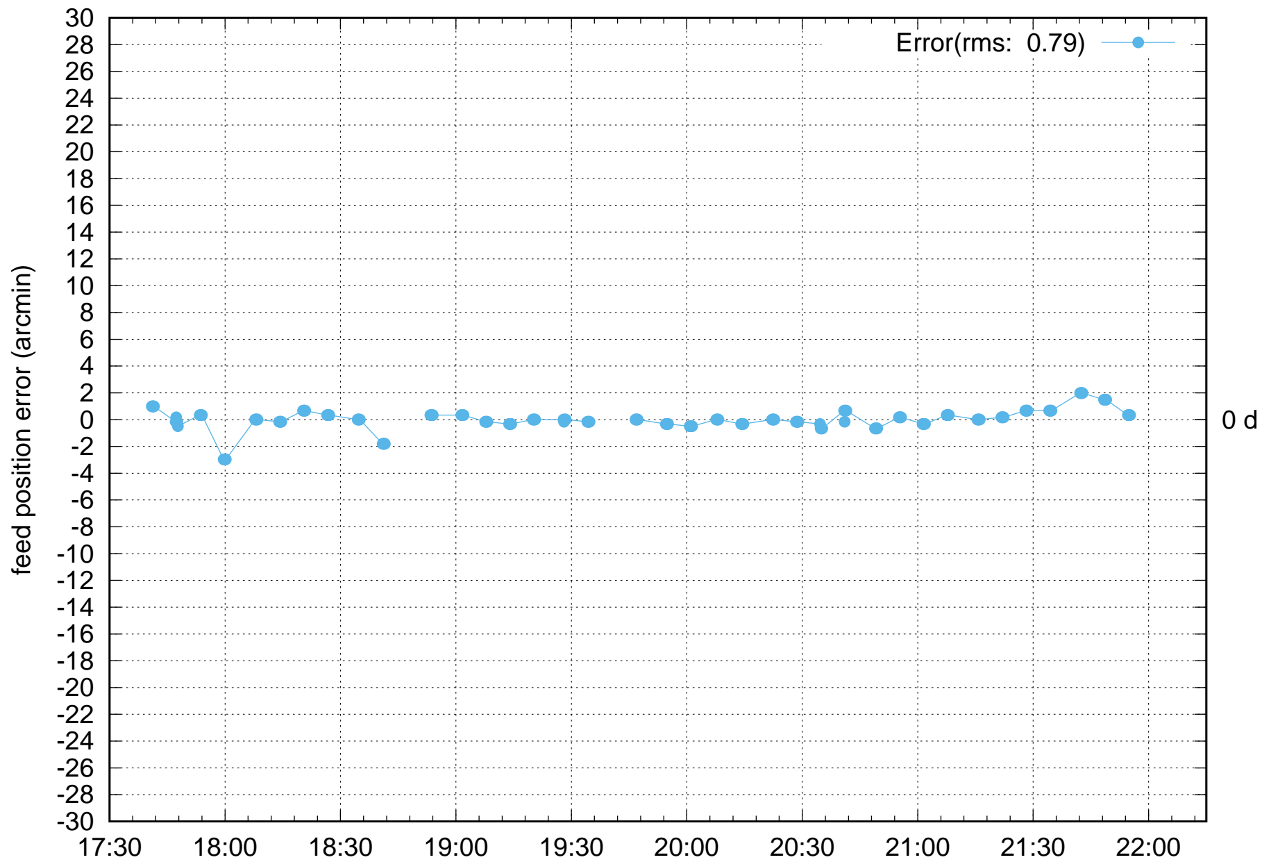
FPS Rotation error: W06-NEW-FPS 08Feb2022
