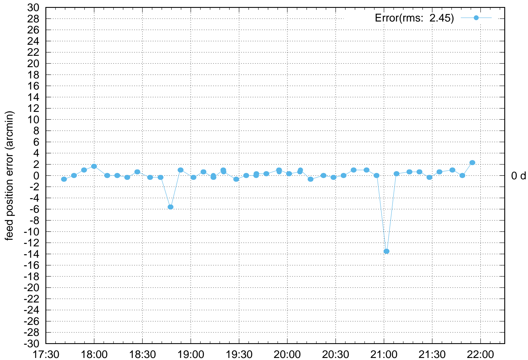
FPS Rotation error: W03-NEW-FPS 08Feb2022
