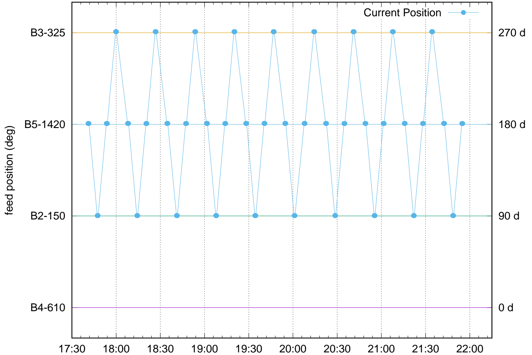
FPS Rotation position: W04-NEW-FPS 08Feb2022
