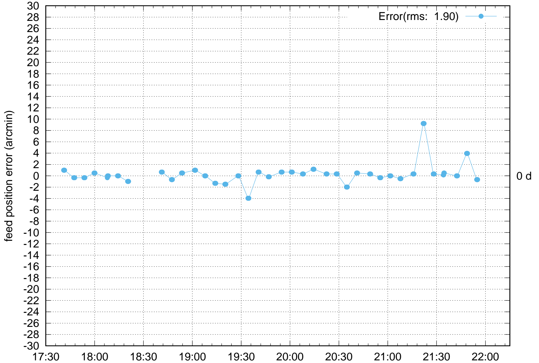
FPS Rotation error: E02-NEW-FPS 08Feb2022
