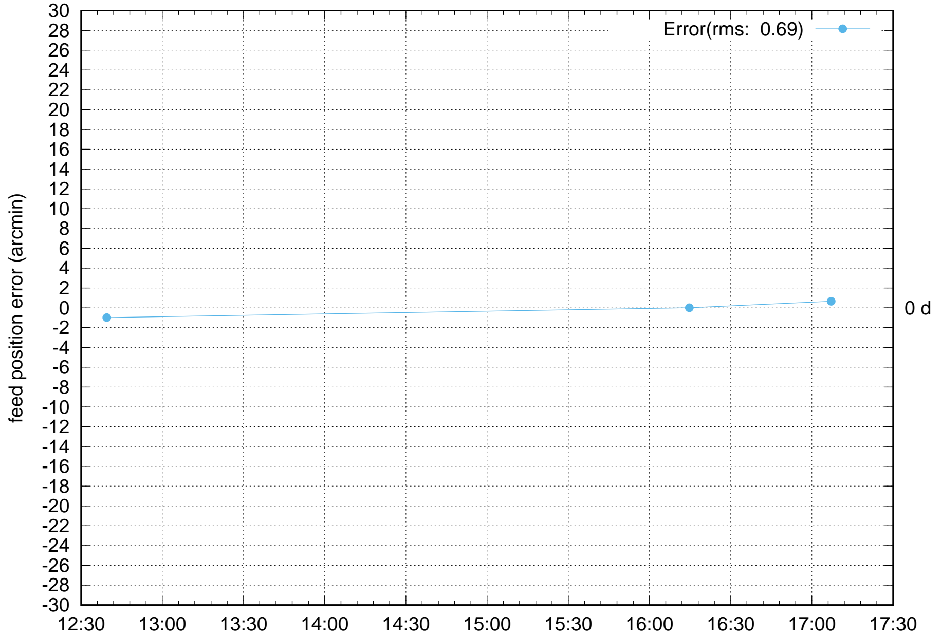
FPS Rotation error: W04-NEW-FPS fps 2 1 mar2022.log
